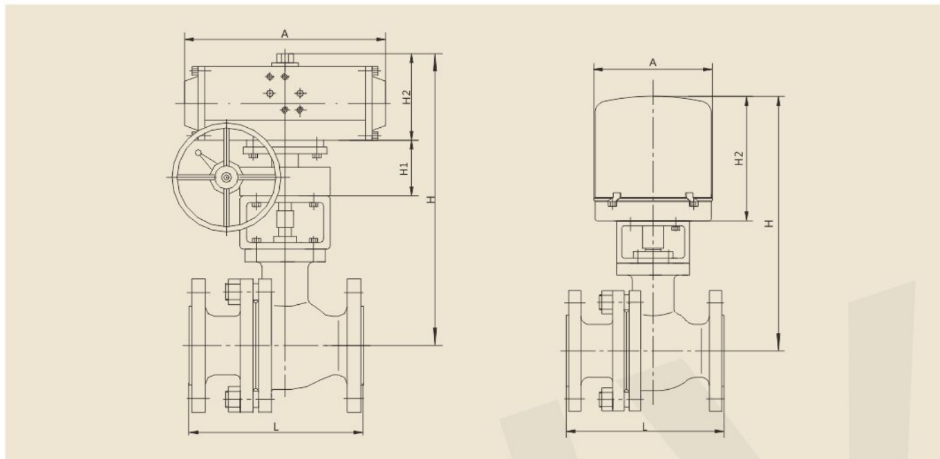
衬氟球阀外形连接尺寸
